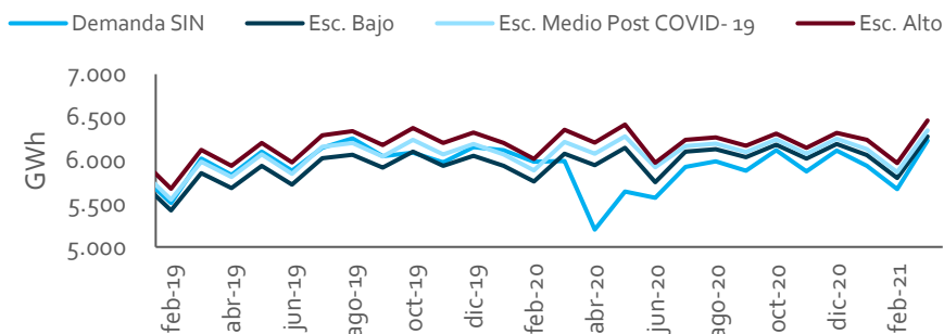
Gráfica 28. Demanda de Energía
