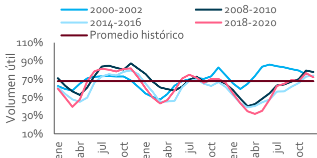
Gráfica 48. Reservas hídricas
