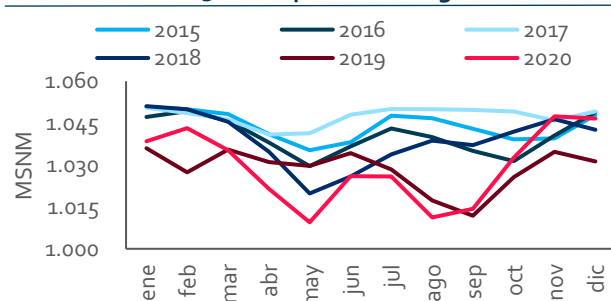
Gráfica 13. Nivel promedio Lago Fortuna
