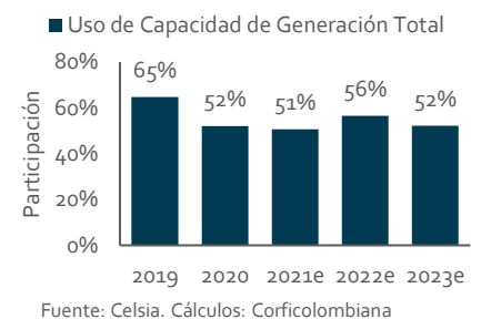
Gráfica 36. Uso de Capacidad
