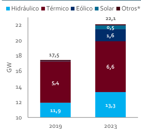
Gráfica 50. Capacidad Efectiva
