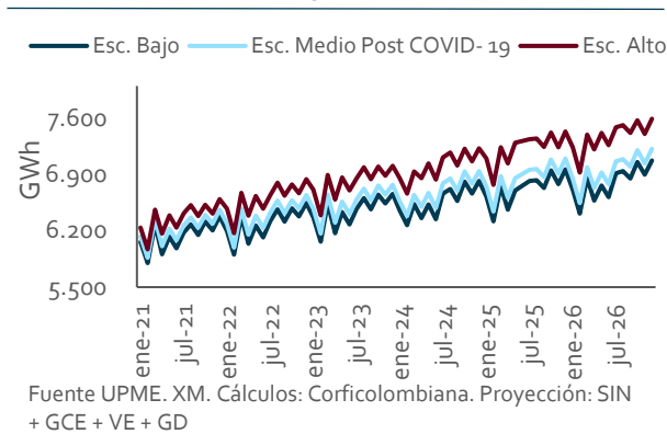
Gráfica 29. Proyección Demanda
