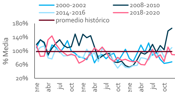
Gráfica 49. Aportes hídricos
