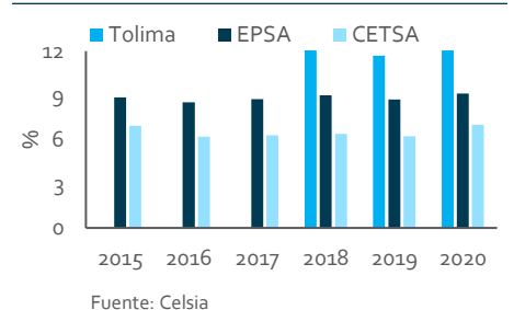
Gráfica 10. Pérdidas de Red
