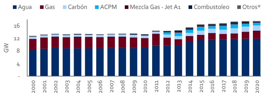
Gráfica 46. Capacidad Efectiva Neta
