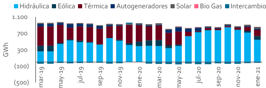
Gráfica 14. Generación Real
