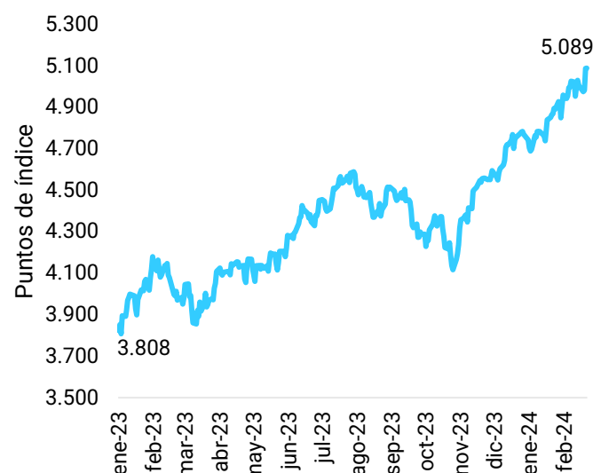
Gráfico 2. Evolución S&P 500
